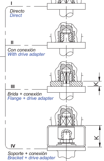
TIPO DE MONTAJE: MOUNTING TYPE:
